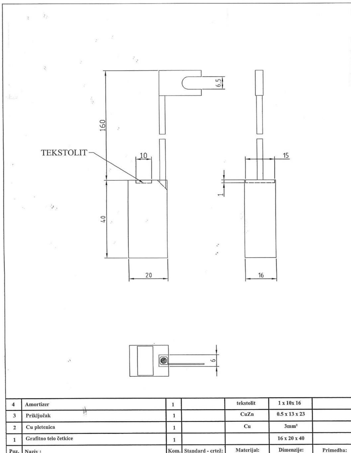
Димензиони цртеж четкице захтеване на позицији бр. 1 – Власинске ХЕ
